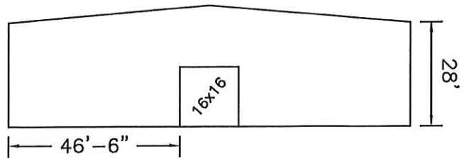
RIGHT ENDWALL
